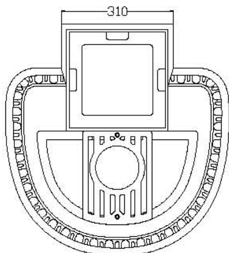
VISTA SUPERIORE
