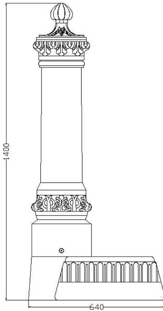
VISTA LATERALE
