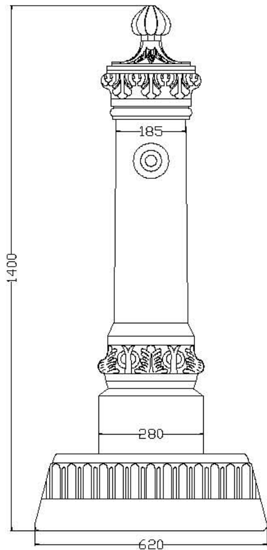
VISTA FRONTALE
